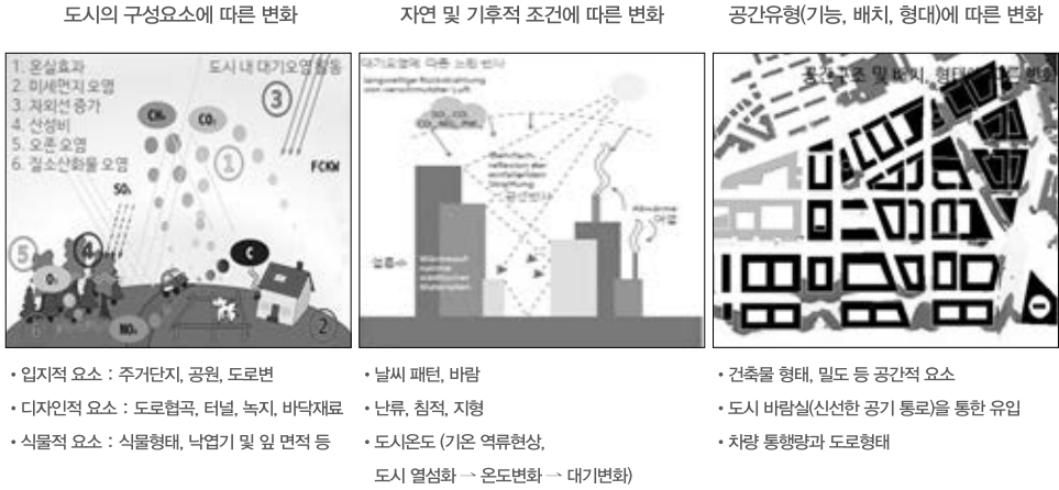
〈그림 3〉 도시 미세먼지의 특성 및 주요내용
