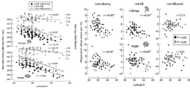
〈그림 9〉 일본의 은행나무와 단풍나무의 단풍 및 낙엽 시기변화
