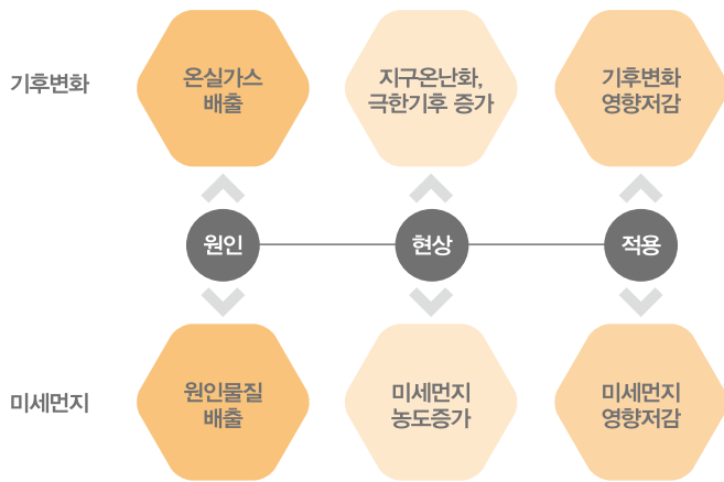
〈그림 7〉 기후변화와 미세먼지 대응 흐름
