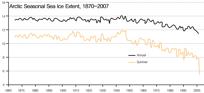
〈그림 3〉 북극 빙산 크기의 연도별 감소
