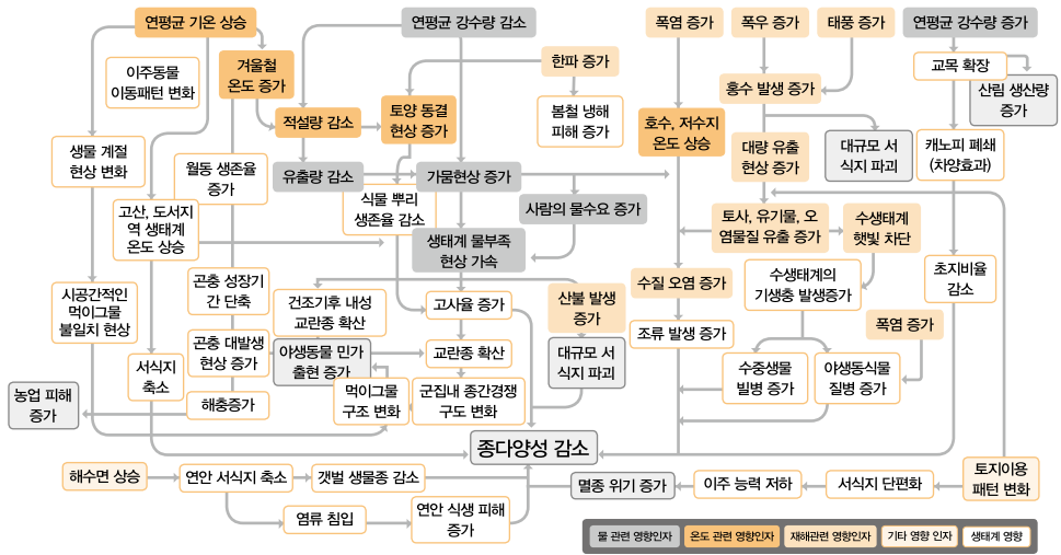
〈그림 1〉 기후변화 요인과 생태계 영향 관계
