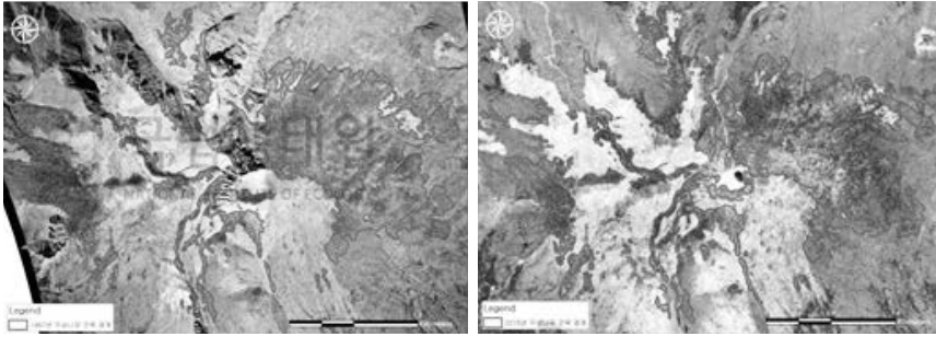
〈그림 14〉 한라산국립공원 내 구상나무 분포 변화(좌: 1967년, 우: 2015년)
