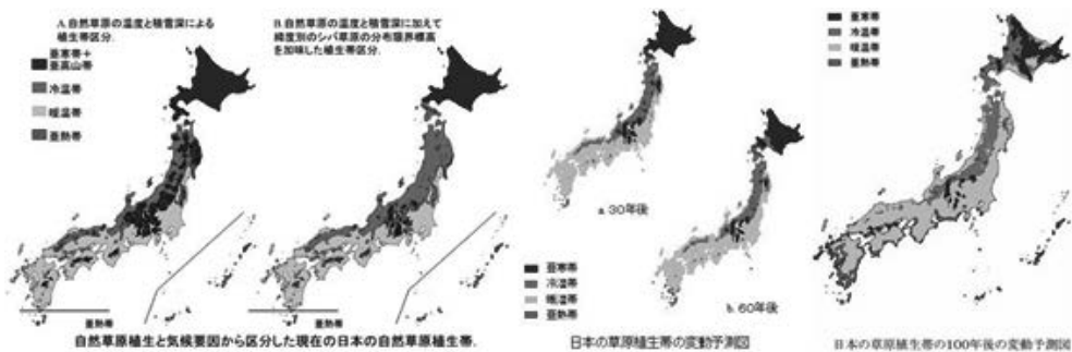
〈그림 4〉 기후변화에 따른 일본 식생대의 변화
