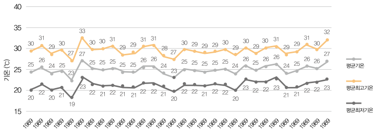
〈그림 3〉 충남지역 2018년 여름(7, 8월) 기온변화
