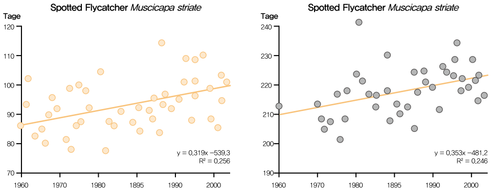
〈그림 11〉 기후변화에 따른 솔딱새류와 대륙검은지빠귀의 번식지 체류시간의 변화
