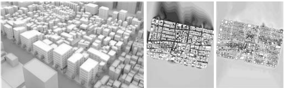
〈그림 2〉 미기후·공간구조에 따른 풍속 및 미세먼지 농도 변화
