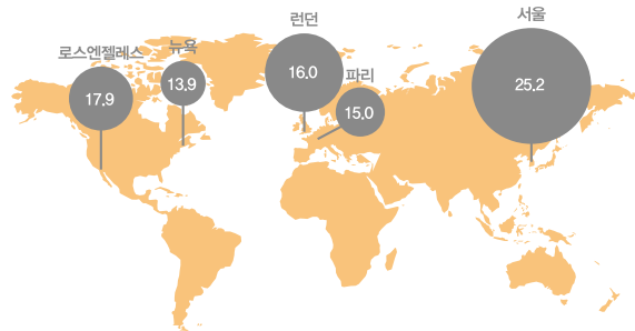
〈그림 5〉 2012년 세계 주요도시 초미세먼지 연평균 농도비교
