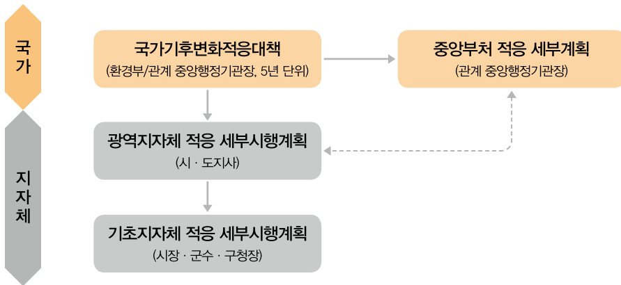
〈그림 2〉 우리나라 기후변화 적응대책 수립·시행 체계
