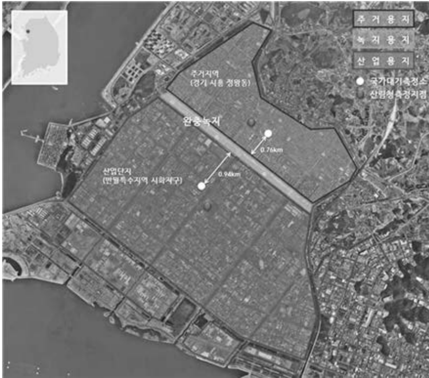
〈그림 5〉 경기도 시흥시 정왕동 및 반월특수지역 시화지구
