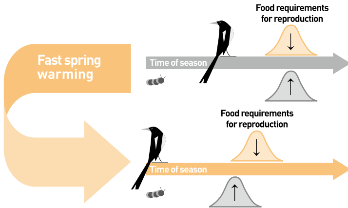
〈그림 6〉 기후변화에 따른 조류의 번식시기와 먹이자원 발생시기의 변화
