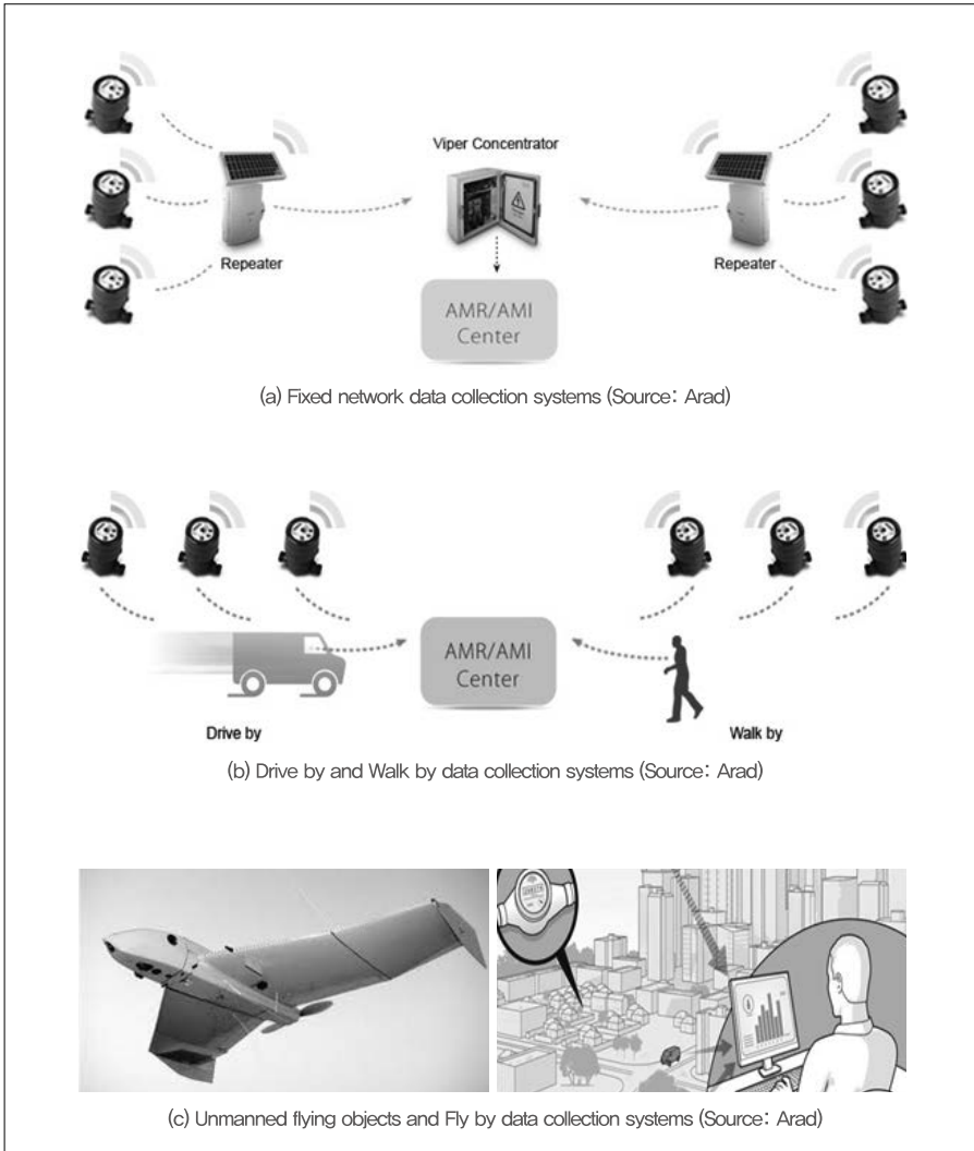
〈그림 4〉 원격검침시스템에서 적용되는 다양한 검침방식
